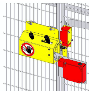
Safe Lock mit Notaus
